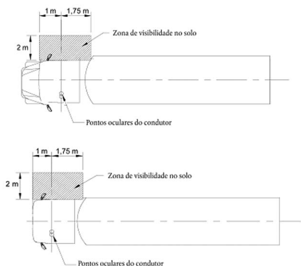
Campo de visão correspondente a espelhos frontais da classe VI
