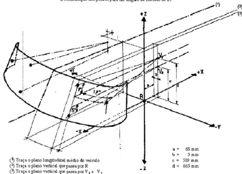
Determinação dos pontos para um ângulo de encosto de 25°
