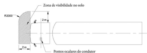
Campo de visão dos dispositivos para visão indireta instalados à retaguarda
