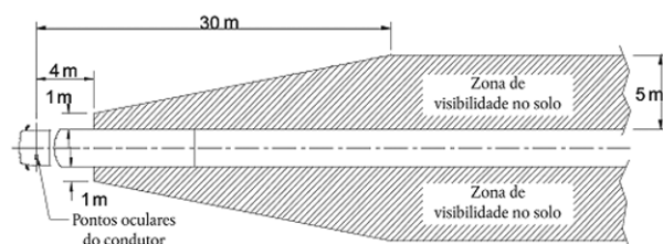
Campo de visão correspondente a espelhos de aproximação da classe V
