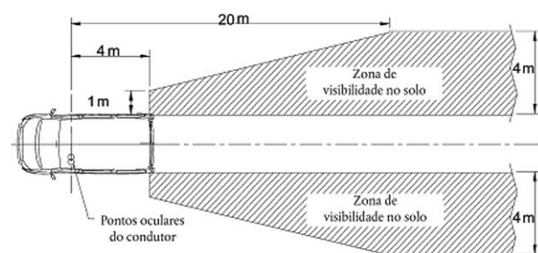
Campo de visão correspondente a espelhos grande angular da classe IV
