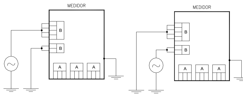
Figura 2a. Ligações a serem feitas para o ensaio de tensão aplicada
