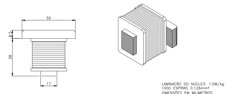
Figura 5 Eletroímã de referência para ensaio da influência da indução magnética CC de origem externa.
