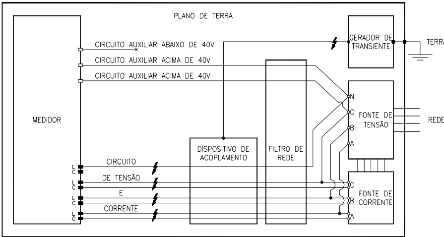
Figura 8b Diagrama de referência das ligações para o ensaio de imunidade a transientes elétricos Aplicação em medidores para conexão diretas.
