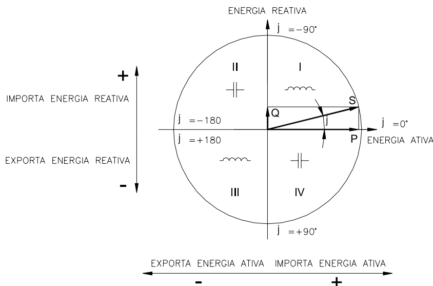
Figura 1 - Representação geométrica das potências ativa e reativa
