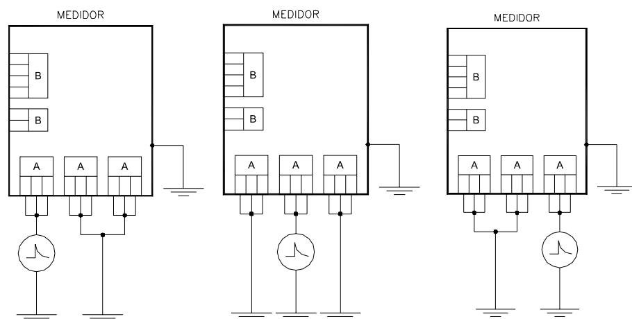
Figura 1a. Ligações a serem feitas para o ensaio de tensão de impulso
