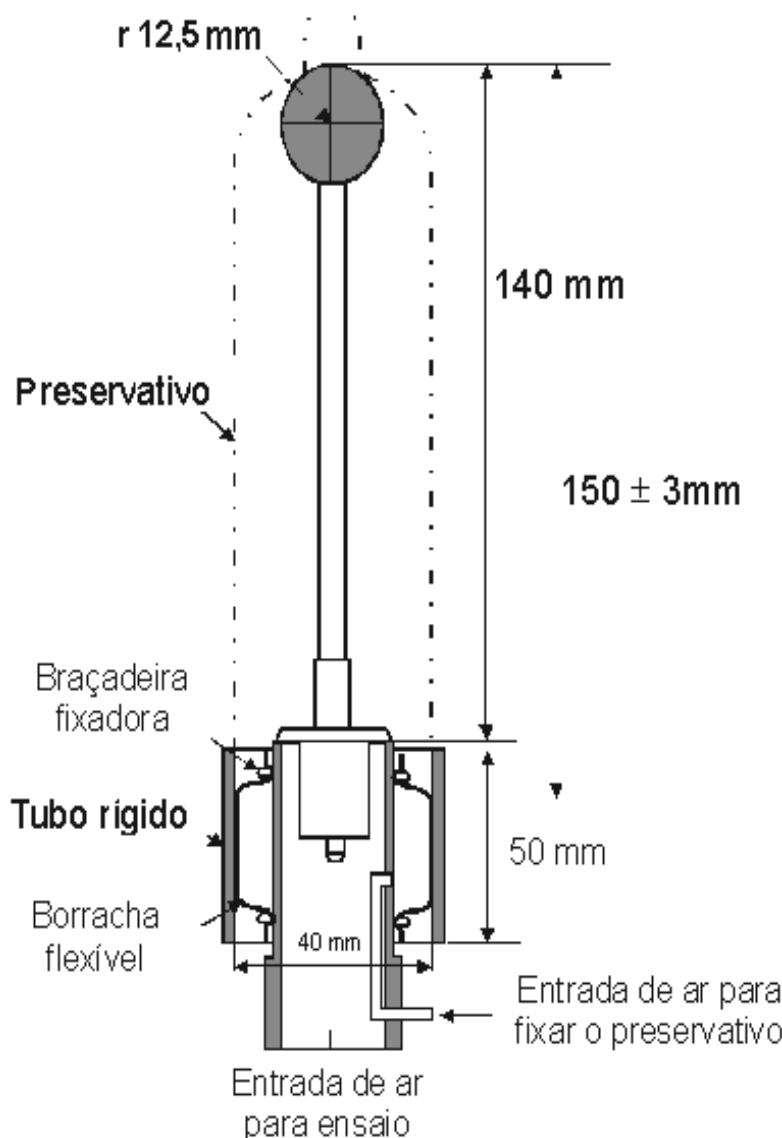
FIGURA 2. Dispositivo para ensaio de capacidade volumétrica e pressão de estouro
