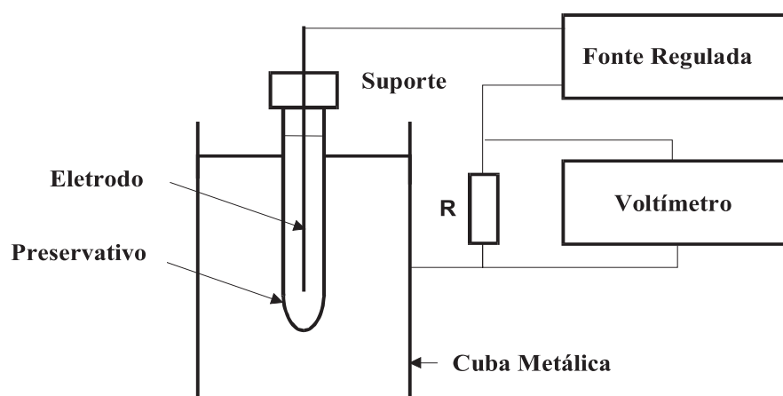
FIGURA 4. Esquema do instrumento para verificação de orifícios
