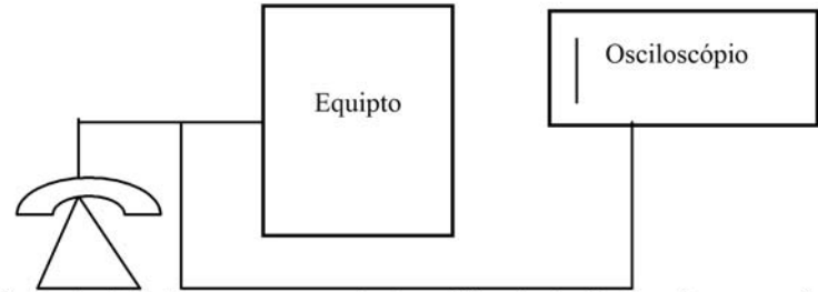
Figura 1 – Montagem para o ensaio de verificação da sinalização para usuários
